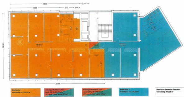
Grundriss 3. Obergeschoss
