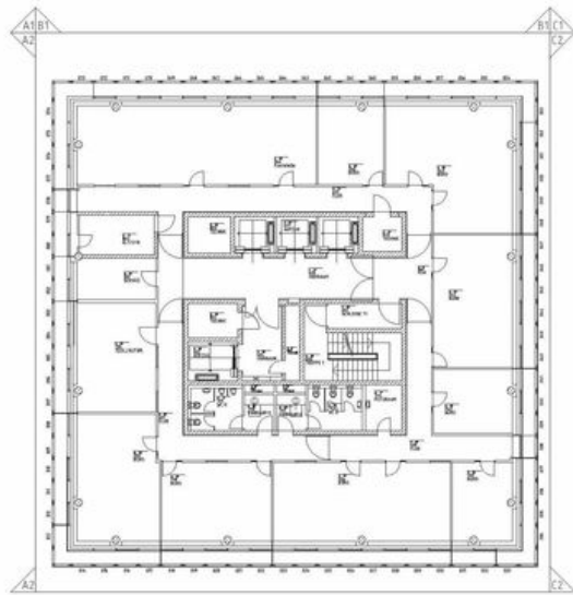
Grundriss 9. Obergeschoss
